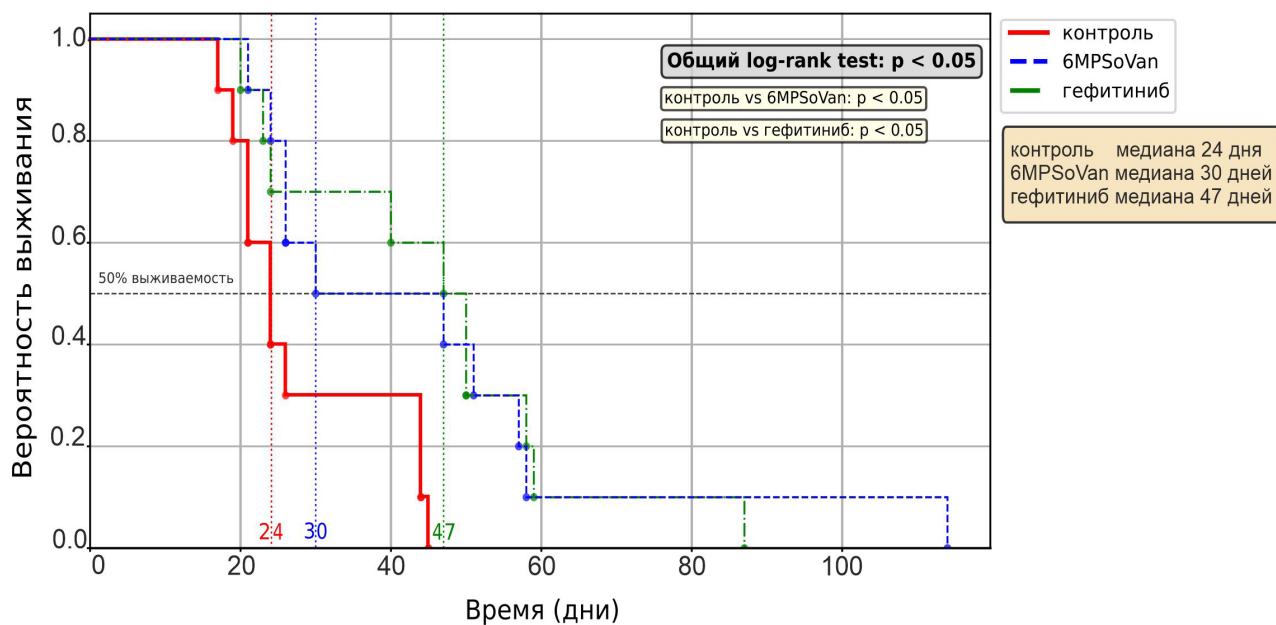
Рис. 2. Кривые общей выживаемости мышей C57BL/6 по методу Каплана — Майера (log-rank-test: \chi^2 = 7.31 , p = 0.025 ). По оси абсцисс — время (дни); по оси ординат — кумулятивная доля выживших
