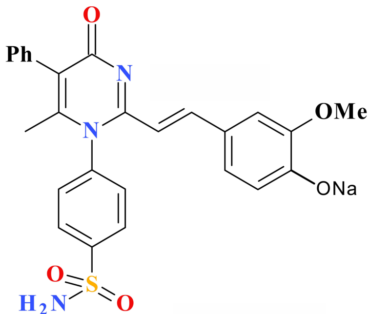
Рис. 1. Структурная формула натриевой соли 4-[2-[2-(4-гидрокси-3-метоксифенил)-винил]-6-метил-4-оксо-5-фенил-4Н-пиримидин-1-ил]-бензсульфамида (6MPSVan-Na)
