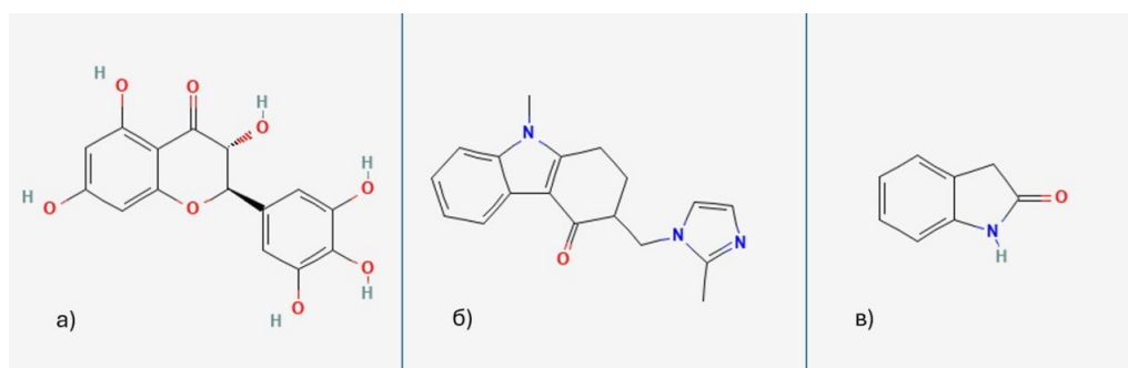
Рис. 3. Химическая структура: 3, а) дигидромирицетина; 3, б) ондансетрона; 3, в) оксиндола.
