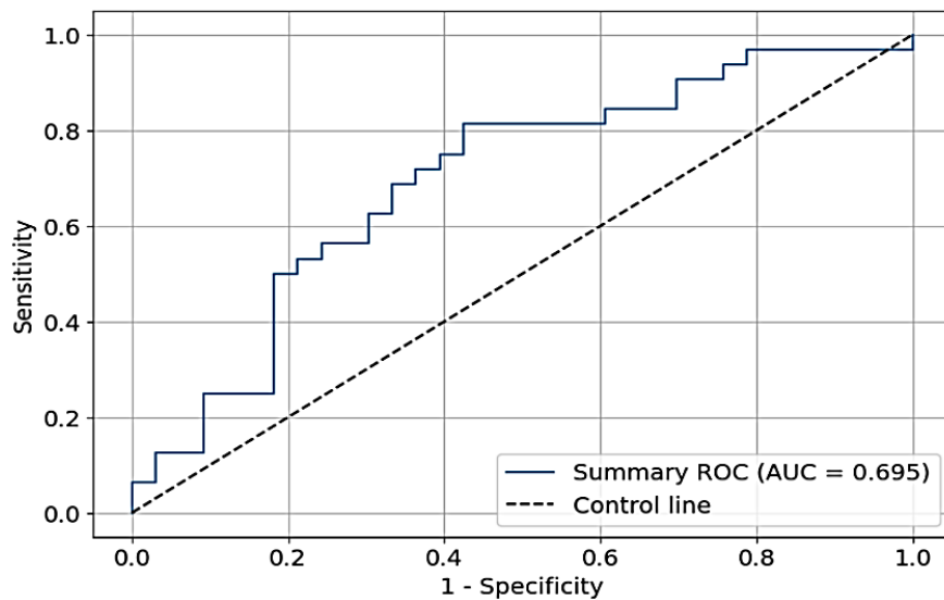
Рис. 3. График ROC-кривой по оценке качества обучения нейросетового классификатора проб выдыхаемого воздуха от пациентов с раком верхних дыхательных путей I–II и III–IV стадий
