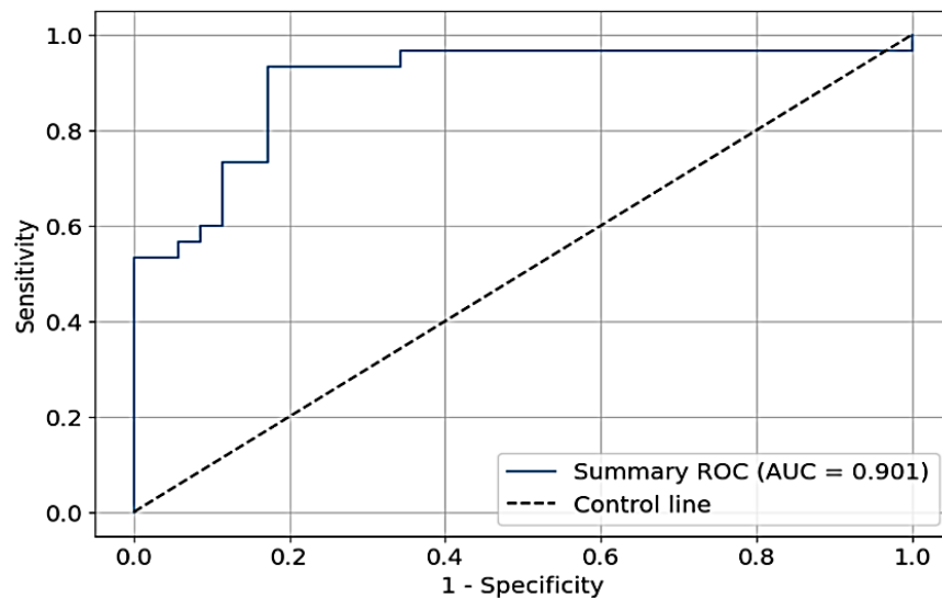
Рис. 1. График ROC-кривой по оценке качества обучения нейросетевого классификатора проб выдыхаемого воздуха от здоровых добровольцев и пациентов с раком верхних дыхательных путей всех (I–IV) стадий Fig. 1. ROC curve analysis of neural network performance for differentiating healthy volunteers from patients with upper respiratory tract cancer (Stages I–IV) using exhaled breath analysis
